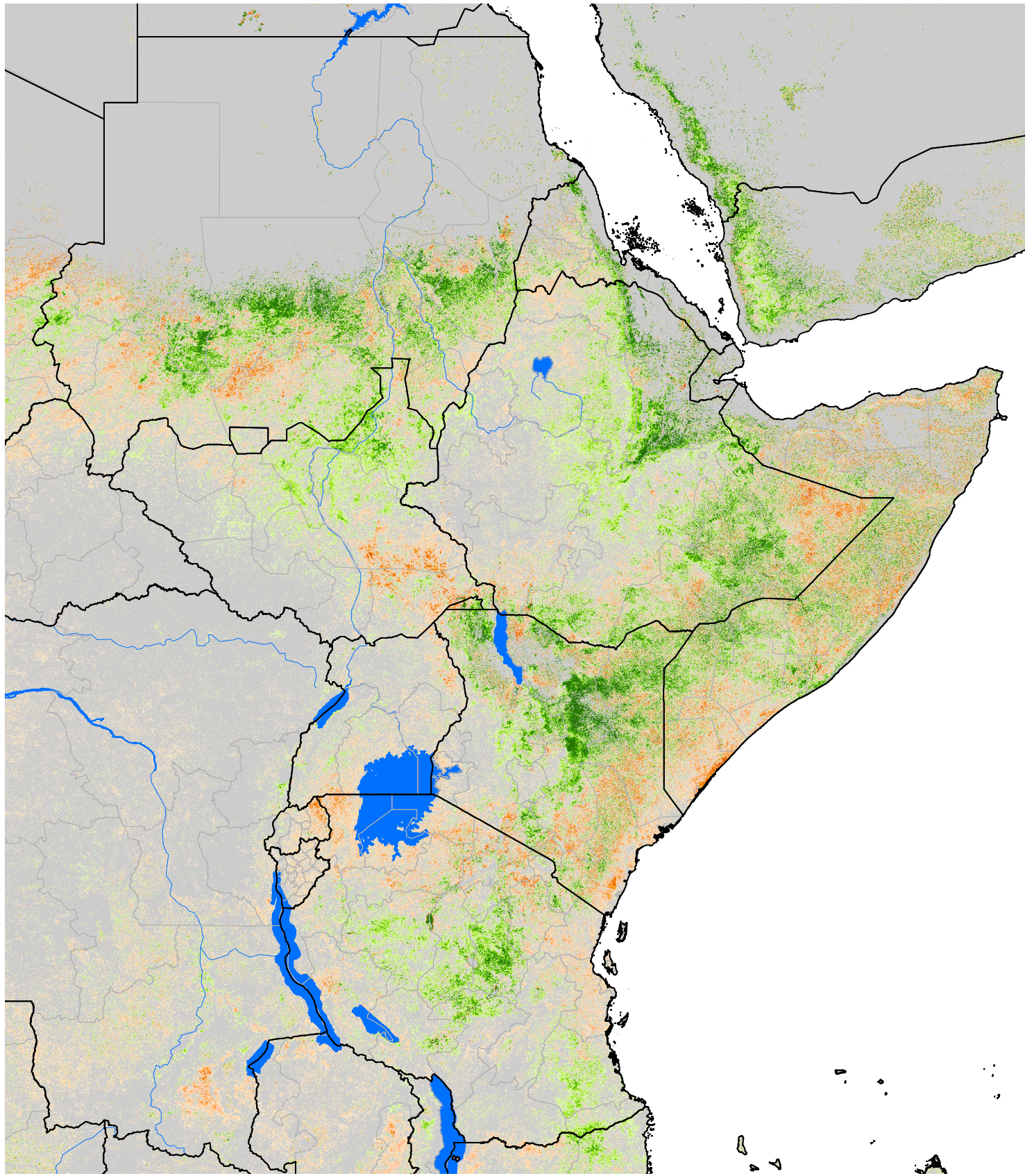
ET Anomaly (%)
